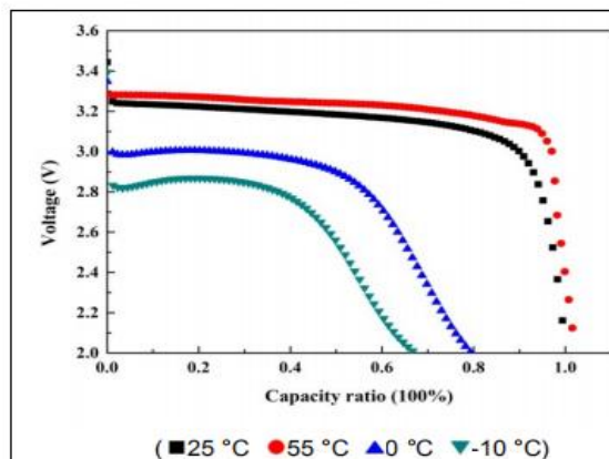
图 1 不同温度下的放电曲线 Fig.1 Discharge curves of different temperature
