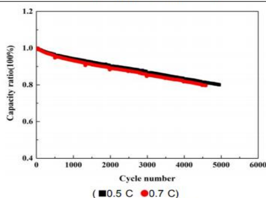
图 4 不同倍率下的循环性能曲线 Fig.4 Cycling performance curves of different rate
