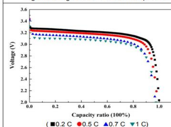
图 3 不同倍率下的放电曲线 Fig.3 Discharge curves of different rate
