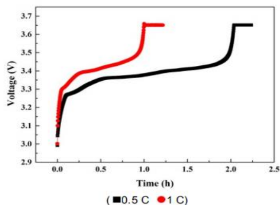
图 2 不同倍率下的充电曲线 Fig.2 Charge curves of different rate
